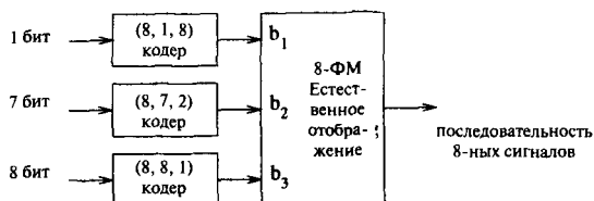
Рис. 114. Пример МСМ системы на сигналах 8-ФМ.
