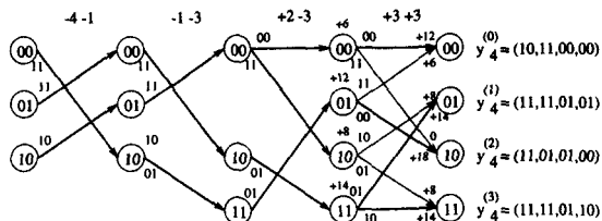
Рис. 72. Работа декодера Витерби с мягким решением на шаге i = 4 .
