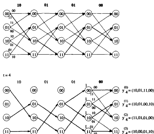
Рис. 43. Операции ВД, Пример 62, шаг 4.
