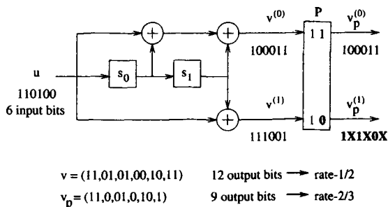
Рис. 50. Кодер перфорированного сверточного кода скорости 2/3 с памятью 2.
