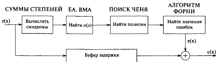
Рис. 21. Архитектура БЧХ декодера.
