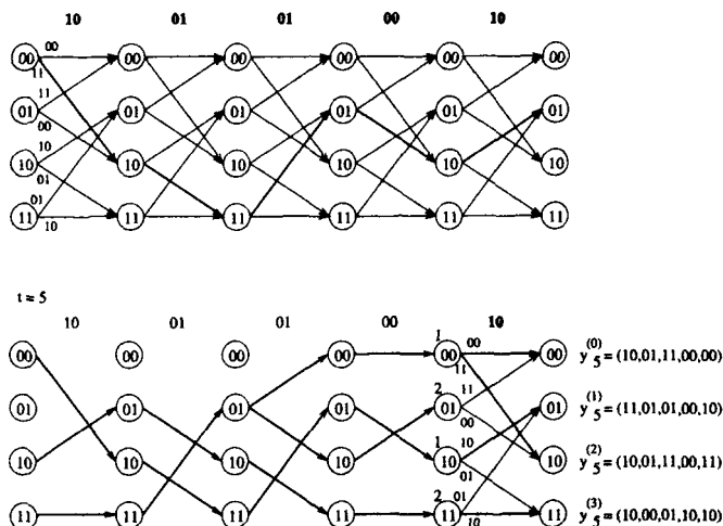
Рис. 44. Операции ВД, Пример 62, шаг 5.
