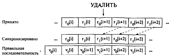
Рис. 46. Пример рассинхронизации ребер декодера Витерби.
