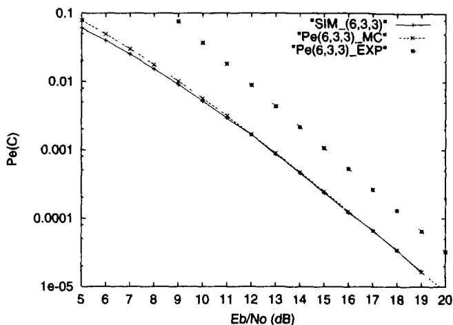
Рис. 13. Двоичная передача по Релеевскому каналу. Результаты моделирования (SIM_(6,3,3)), оценка границы объединения методом Монте-Карло ( P_e(6,3,3)_{MC} ) и граница Чернова ( P_e(6,3,3)_{EXP} ) для двоичного (6,3,3) кода.
