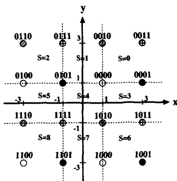
Рис. 113. 16-КАМ созвездие для практической ТСМ с двухуровневым декодированием.
