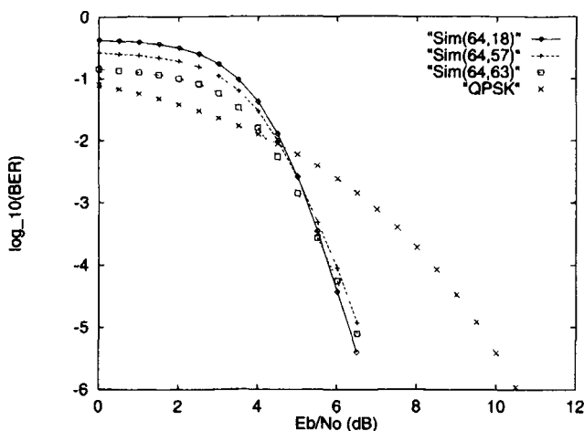
Рис. 120. Результаты моделирования трехуровневой кодовой модуляции на сигналах 8-ФМ с разбиениями по схеме Унгербёка.
