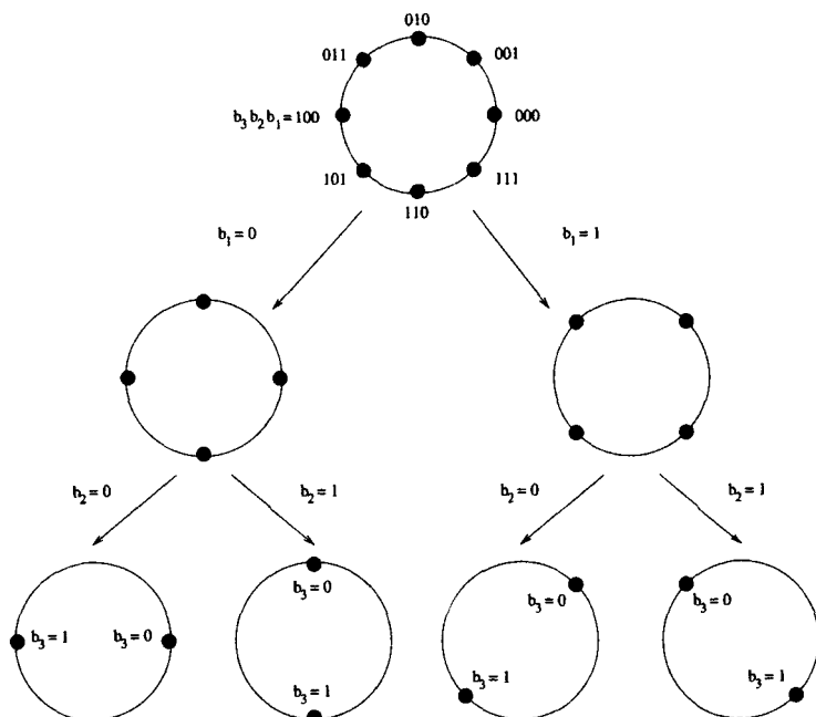
Рис. 103. Естественное отображение для 8-ФМ созвездия.
