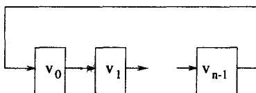
Рис. 16 Циклический регистр сдвига
