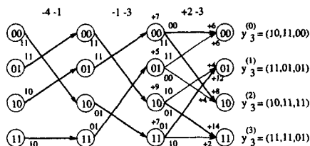
Рис. 71. Работа декодера Витерби с мягким решением на шаге i = 3 .
