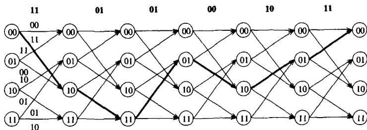
Рис. 68. Путь на треллисе, соответствующий последовательности u = (110100) .
