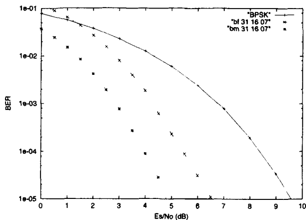
Рис. 92. Эффективность алгоритмов Берлекэмпа-Мэсси и BF-алгоритма Галлагера для двоичного (31, 16, 7) БЧХ кода.
