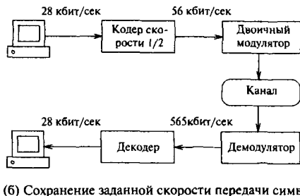
Рис. 96 Эффект кодирования для двоичной системы передачи информации.
