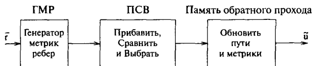
Рис. 39. Структурная схема декодера Витерби.
