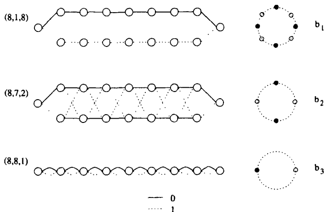
Рис. 115. Решетки компонентных кодов в примере МСМ на сигналах 8-ФМ.
