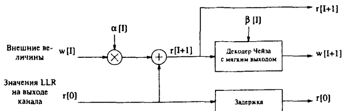
Рис. 85. Блок схема декодера Чейза с мягким выходом.
