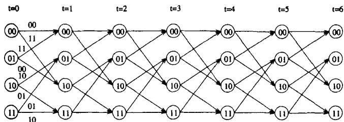
Рис. 32. Шесть секций решетчатой диаграммы сверточного кода скорости 1/2 и памяти 2.
