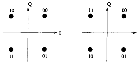
(а) Отображение Грея (б) Естественное отображение
