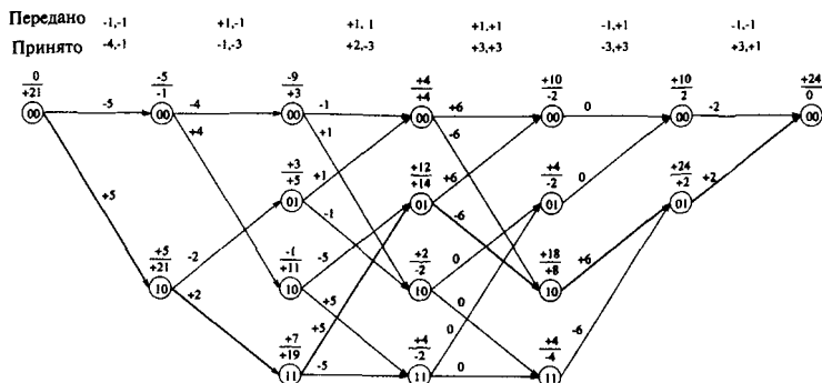
Рис. 77. Решетчатая диаграмма, использованная для SOVA декодирования в Примере 88.
