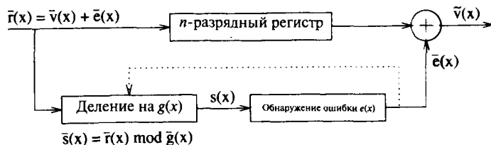
Рис. 18. Обобщенная структура декодера циклического кода.
