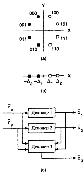
Рис. 121. 8-ФМ созвездие с блоковым разбиением: (а) нумерация, (б) проекции на X координату, (в) структура декодера ( c_i обозначают оценки кодовых слов в коде C_i , i = 1, 2, 3 ).
