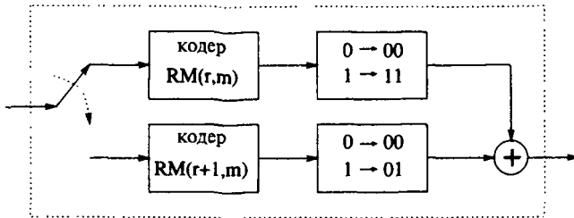
Рис. 66. Кодер двоичного RM(r+1, m+1) кода в виде двухуровневого ОКК.
