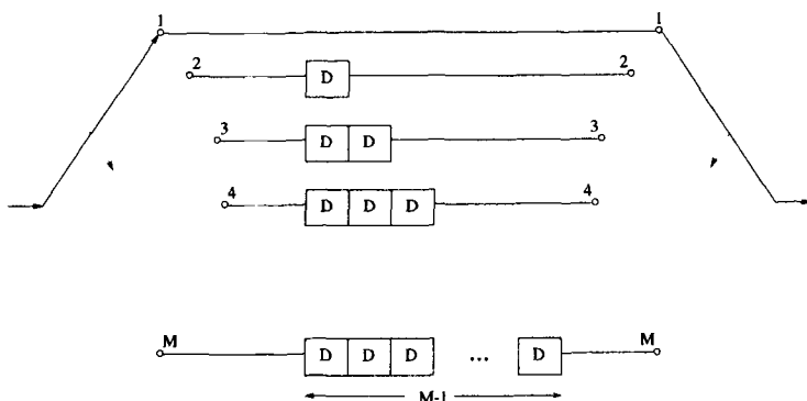
Рис. 63. Сверточный интерливер.
