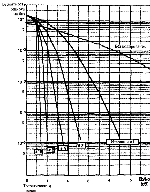
Рис. 78. Вероятность ошибки турбо кода скорости 1/2 с компонентными RSC кодами скорости 2/3, памяти 4, g_0 = 21 и g_1 = 37 , и блоковым перемежителем размера 256 \times 256 = 65536 . Скопировано из [BG2] с разрешения IEEE (©1996 IEEE).
