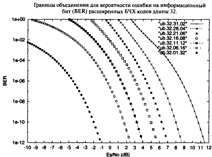
Рис. 26. Оценки BER по границе объединения для расширенных БЧХ кодов длины 32. Двоичный канал с АБГШ.
