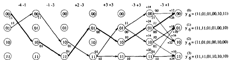
Рис. 74. Работа декодера Витерби с мягким решением на шаге i = 6 .
