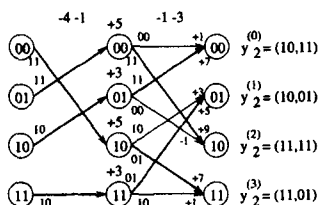
Рис. 70. Работа декодера Витерби с мягким решением на шаге i = 2 .
