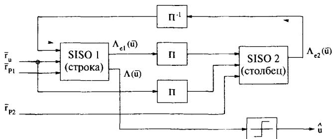
Рис. 82. Структурная схема итеративного декодера для параллельного составного (каскадного) кода.
