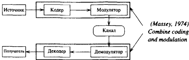
Рис. 100. Идея совместного кодирования и модуляции.
