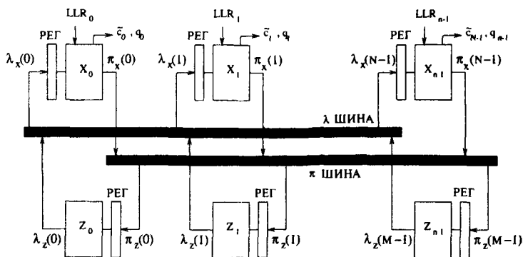
Рис. 94. Параллельная архитектура IBP декодера.
