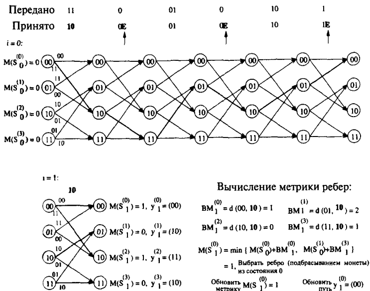
Рис. 51. Работа декодера Витерби для перфорированного кода (РСС) скорости 2/3, памяти 2, i = 1 .
