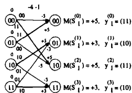
Рис. 69. Работа декодера Витерби с мягким решением на шаге i = 1 .
