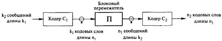
Рис. 55. Кодер двумерного кода-произведения с блоковым перемежителем (интерливером).
