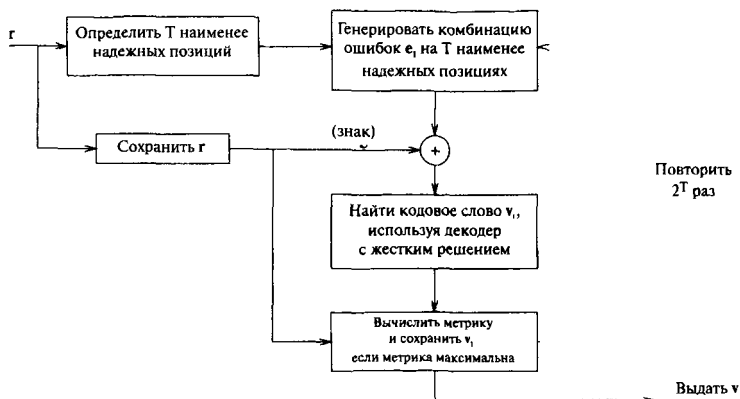
Рис. 76. Структурная схема алгоритма Чейза, Тип -II.
