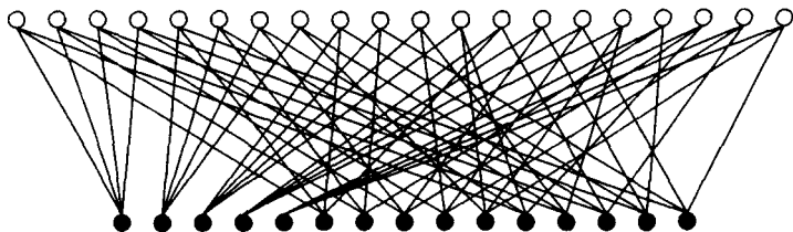
Рис. 87. Граф Таннера для кода Галлагера (20, 5).
