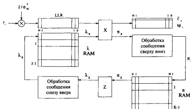
Рис. 95. Последовательная архитектура IВР декодера.
