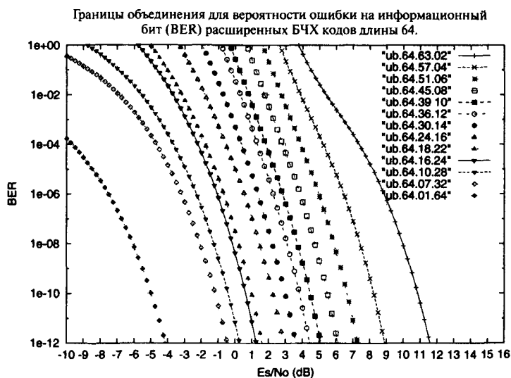
Рис. 27. Оценки BER по границе объединения для расширенных БЧХ кодов длины 64. Двоичный канал с АБГШ.
