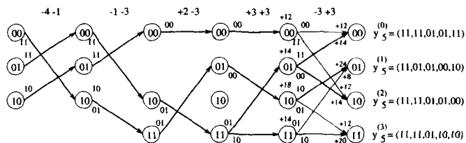
Рис. 73. Работа декодера Витерби с мягким решением на шаге i = 5 .
