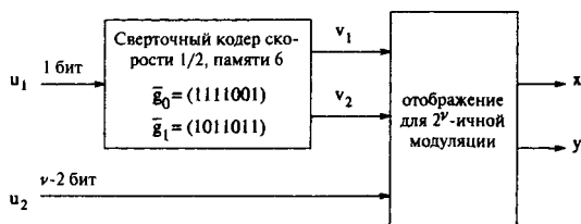
Рис. 109. Структурная схема кодера практической конструкции TCM.
