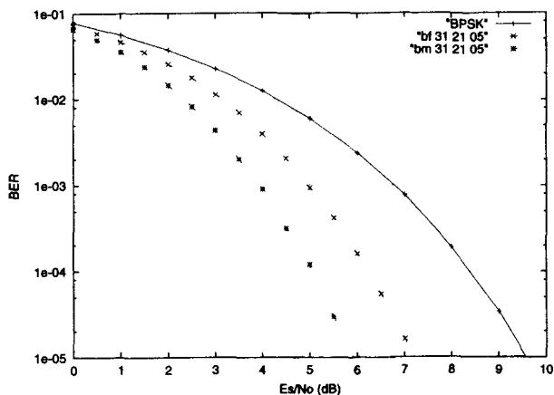
Рис. 91. Эффективность алгоритмов Берлекэмпа-Мэсси и BF-алгоритма Галлагера для двоичного (31, 21, 5) БЧХ кода.
