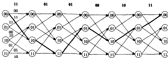
Рис. 33. Путь на треллисесверточного кода скорости 1/2 и памяти 2.
