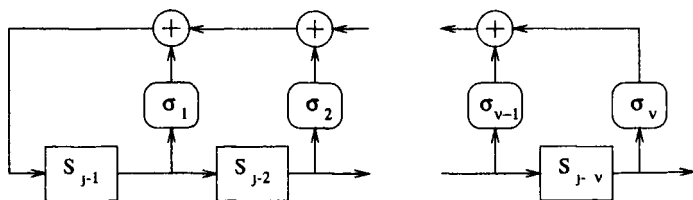
Рис. 23. ЛПРОС с отводами \sigma_1, \sigma_2, \dots, \sigma_v и выходом S_1, S_2, \dots, S_{2v} .
