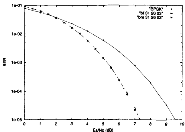
Рис. 90. Эффективность алгоритмов Берлекэмпа-Мэсси и BF-алгоритма Галлагера для двоичного (31, 26, 3) БЧХ кода.
