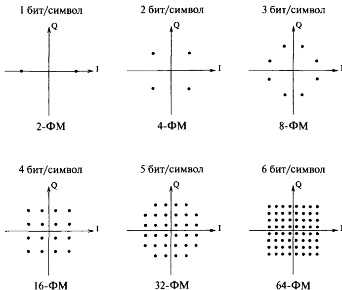
Рис. 97. Примеры M -ФМ и M -КАМ сигнальных созвездий.
