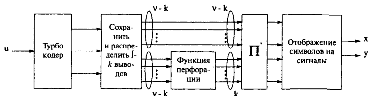
Рис. 124. Комбинация турбо кода и цифровой модуляции [LGB].
