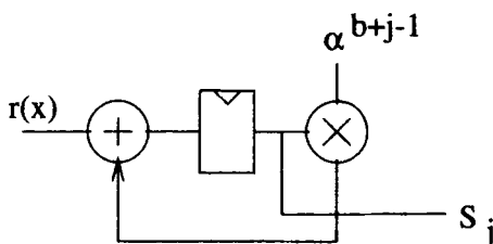
Рис. 22. Пример схемы вычисления синдрома.
