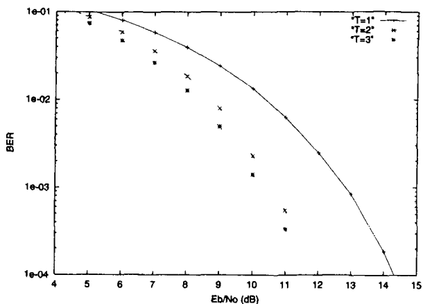
Рис. 88. Характеристики кода Галлагера (20, 5) для алгоритма с перевертыванием бита. Четыре итерации с различными порогами.
