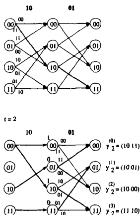
Рис. 41. Диаграмма вычислений декодера Витерби, Пример 62 , шаги i = 2 .
