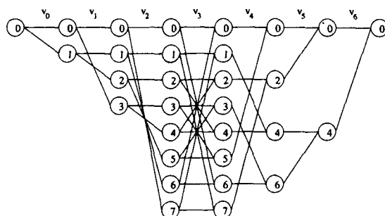
Рис. 75. Решетка кода Хемминга (7, 4, 3).
