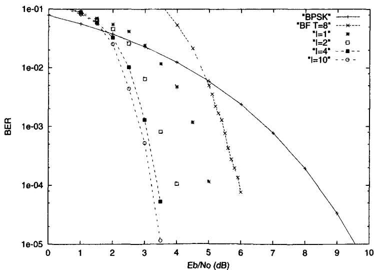
Рис. 93. Эффективность итеративного декодирования двоичного (273, 191) кода.
