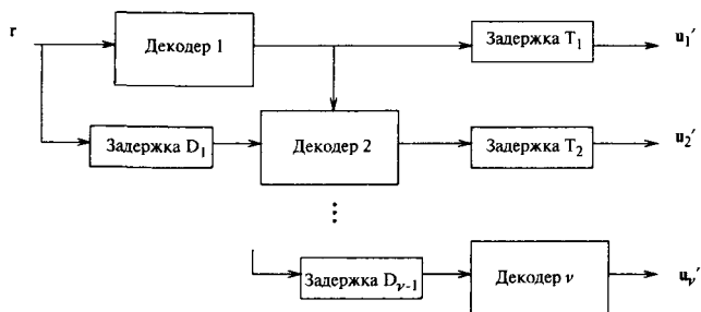
(б) Многоступенчатый декодер
