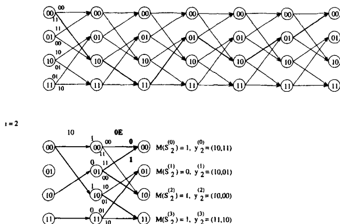
Рис. 52. Работа декодера Витерби для РСС скорости 2/3 и памяти 2, шаг i = 2 .
